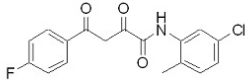
PC-3572501, DMSO-d6
